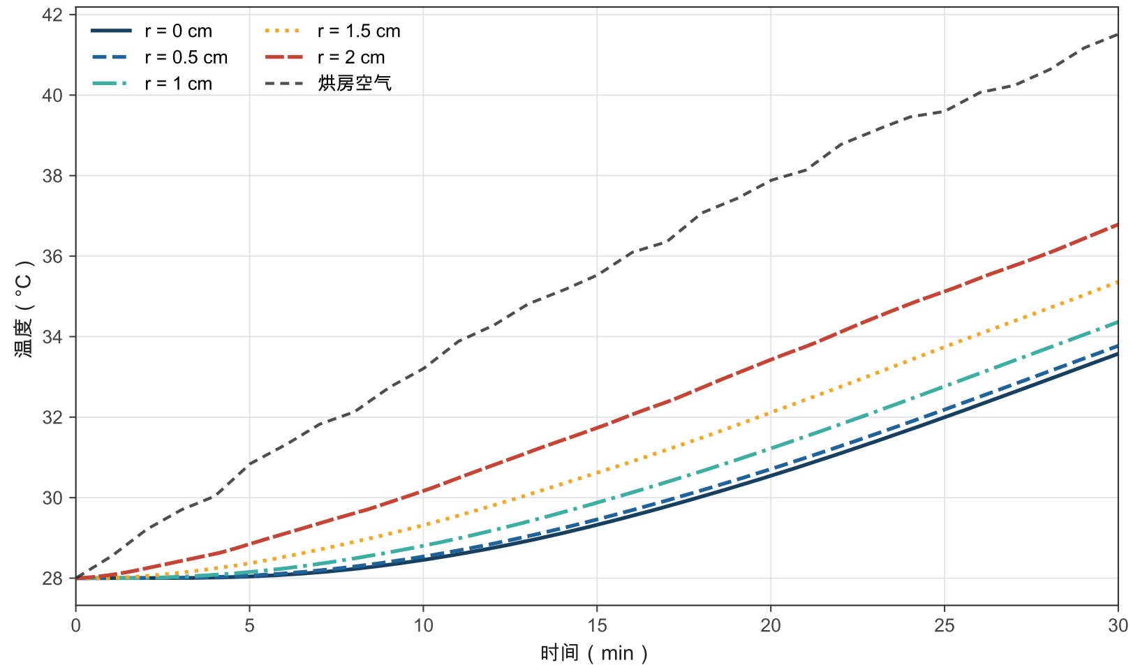
不同径向位置的温度随时间变化
