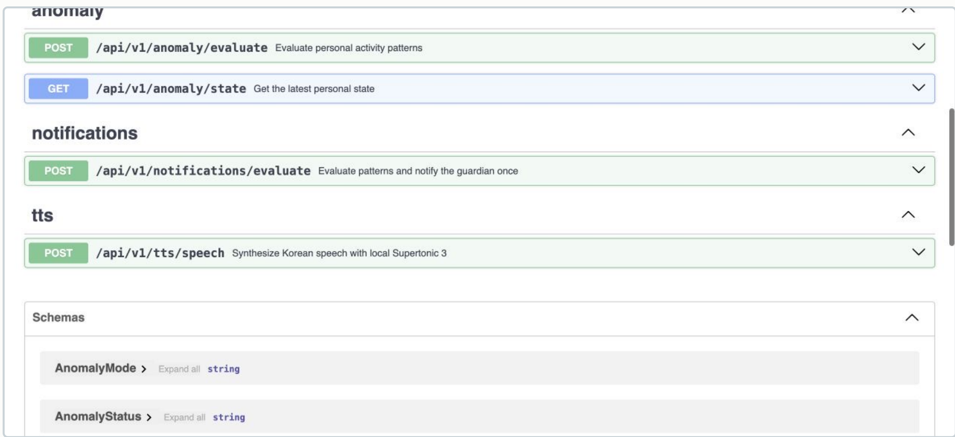
그림 2. 로컬 실행 화면. anomaly, notification, Supertonic 3 TTS endpoint가 OpenAPI 3.1 문서에 등록되어 있다.
