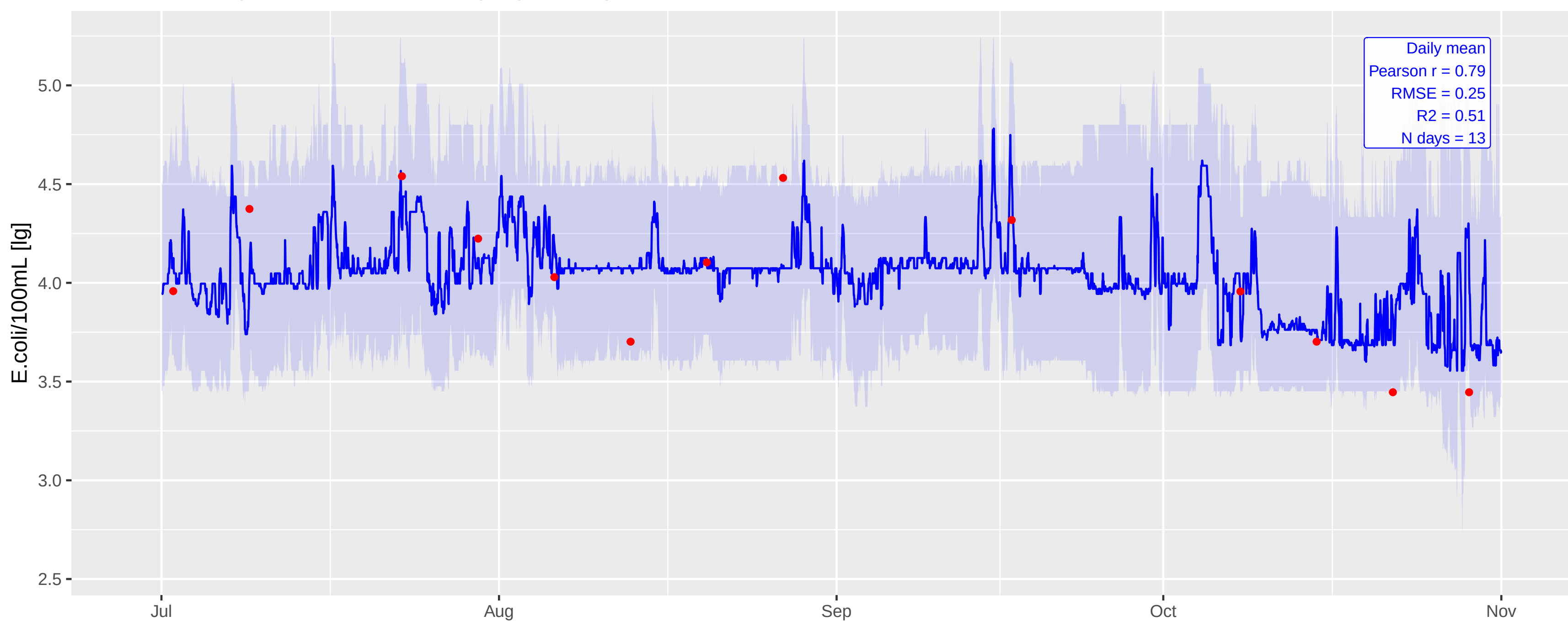
Labormessung vs Modellvorhersage (bestR2)
