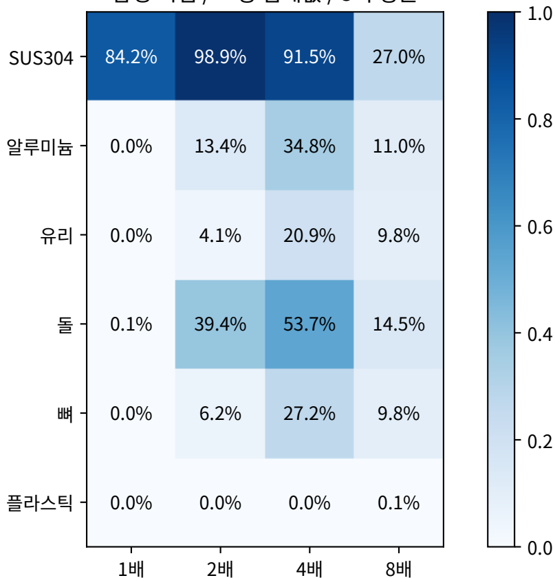
MAL+UQ: 재질·크기별 정보 도달률 합성 시험 / 고정 임계값 / 3회 평균
