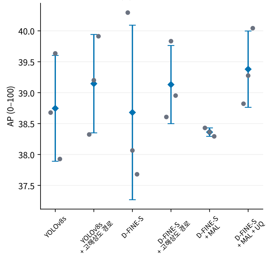
(a) 평균 정밀도
