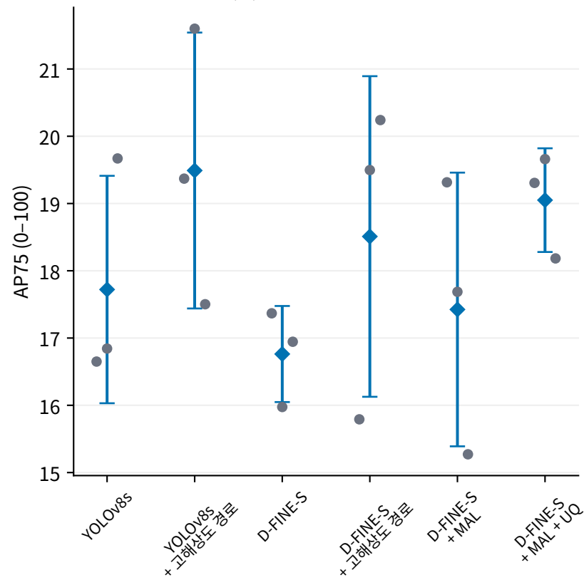
(b) 정밀한 위치 검출
