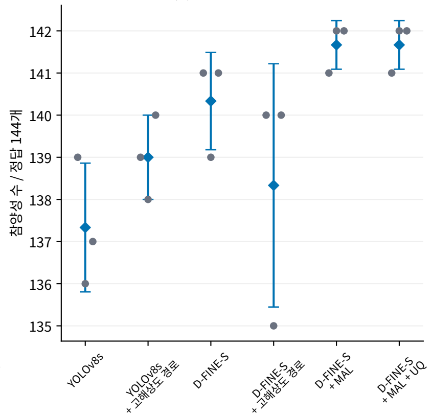
(c) 오탐 예산 내 검출
