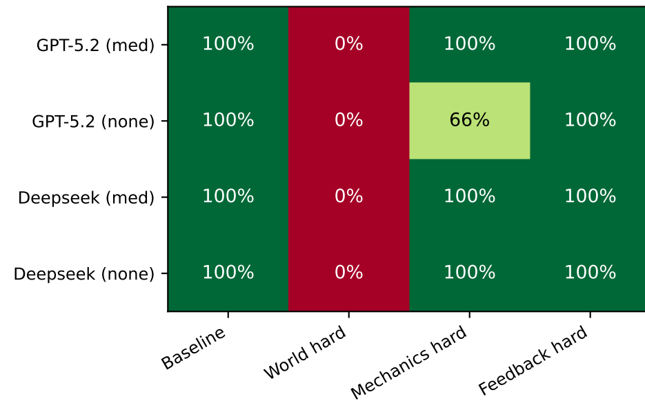
BP35
