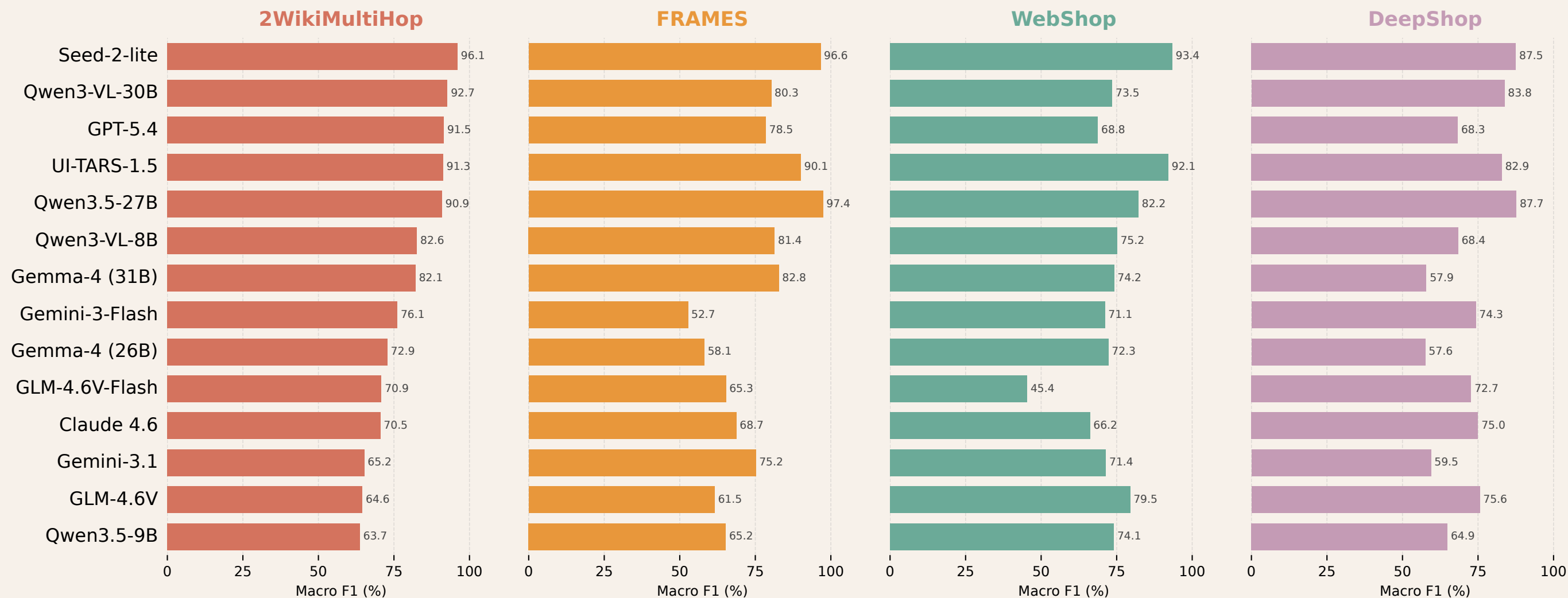
A. Closed-set Attribution — Macro F1 (%) ↑
