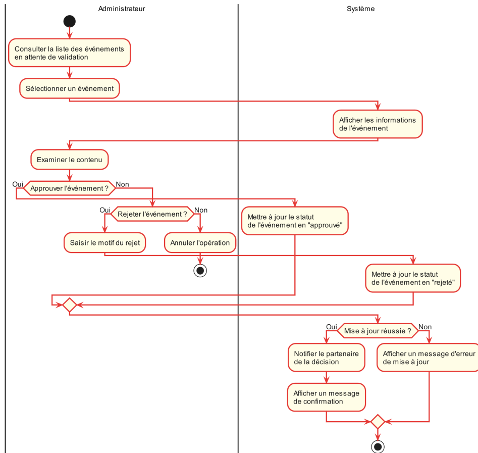
FIGURE 1.7 – Diagramme d'activité du contrôle de l'offre événementielle
