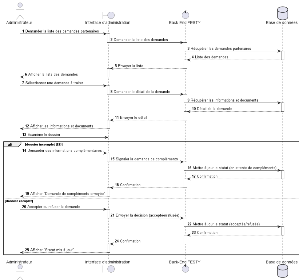
FIGURE 1.4 – Diagramme de séquence du scénario de traitement d'une demande partenaire
