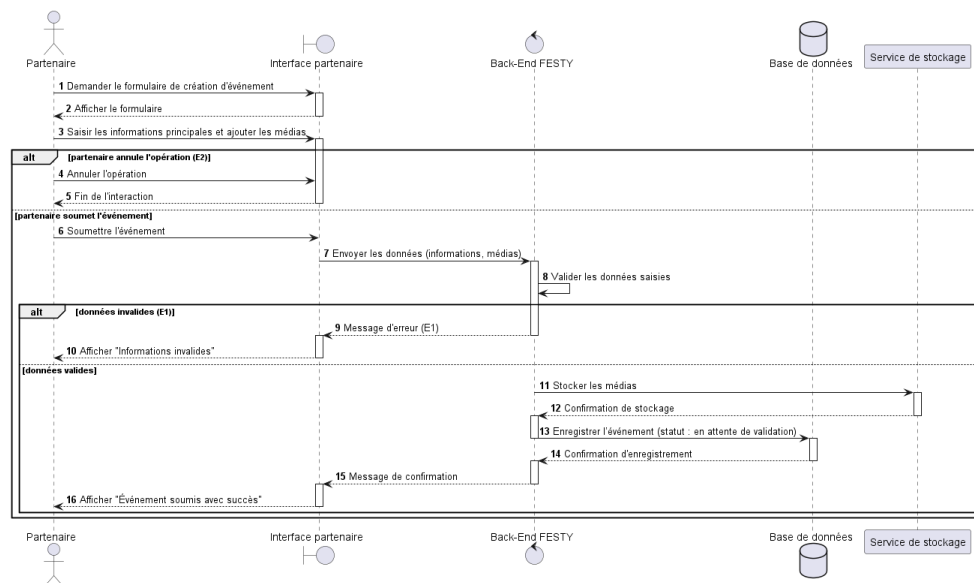
FIGURE 1.6 – Diagramme de séquence du scénario de création d'un événement
