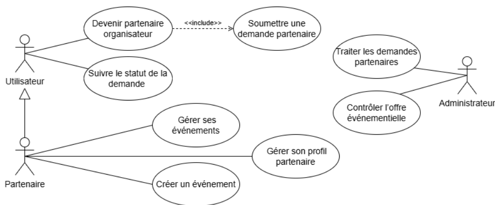
FIGURE 1.1 – Diagramme de cas d'utilisation du Sprint 2
