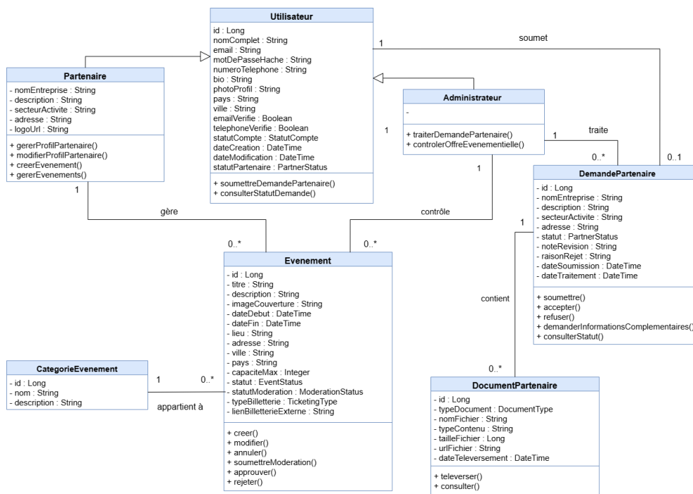
FIGURE 1.2 – Diagramme de classes du Sprint 2
