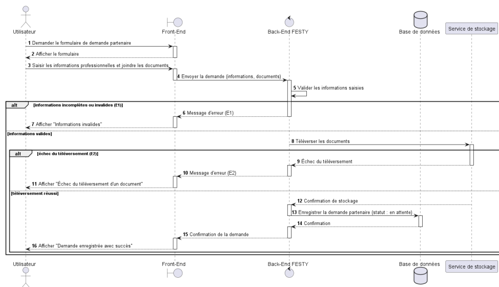
FIGURE 1.3 – Diagramme de séquence du scénario de soumission d'une demande partenaire
