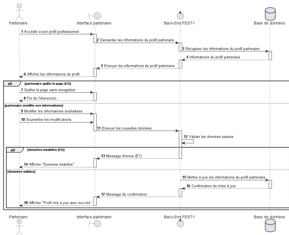
FIGURE 1.5 – Diagramme de séquence du scénario de gestion du profil partenaire
