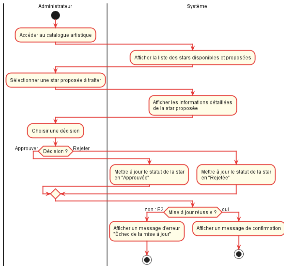
FIGURE 1.7 – Diagramme d'activité du scénario de gestion du catalogue artistique
