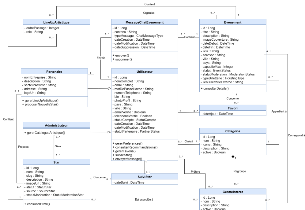
FIGURE 1.2 – Diagramme de classes du Sprint 3
