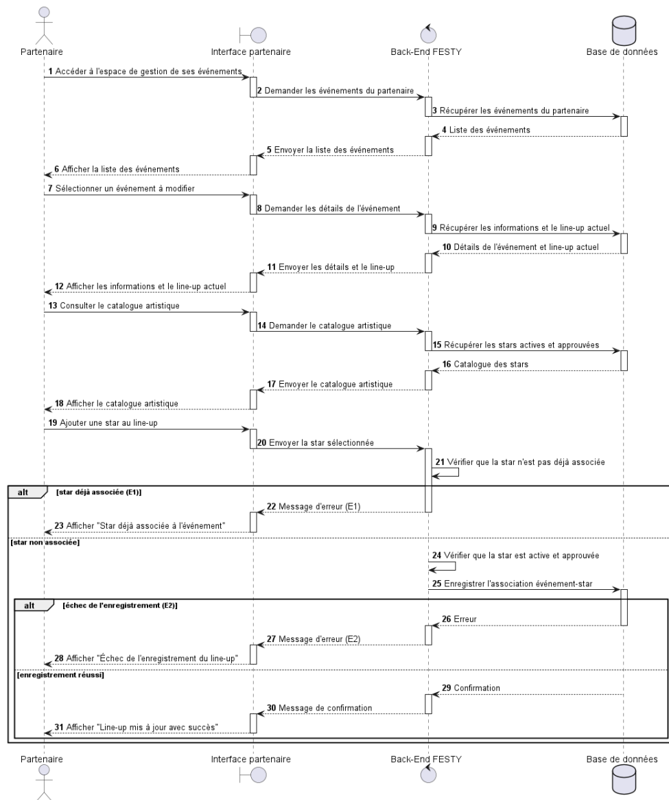
FIGURE 1.5 – Diagramme de séquence du scénario de gestion du line-up artistique
