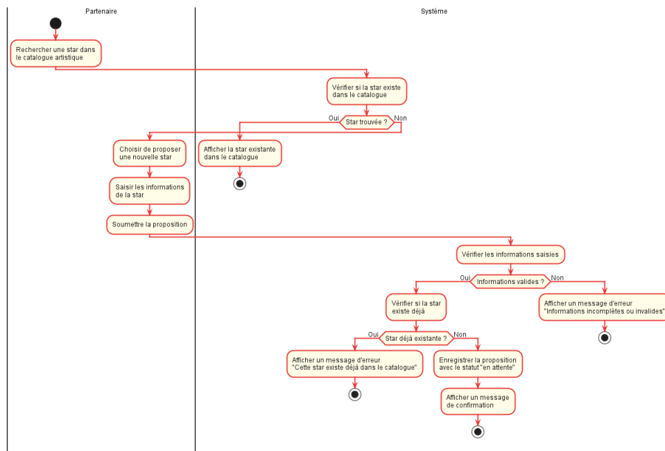
FIGURE 1.6 – Diagramme d'activité du scénario de proposition d'une nouvelle star
