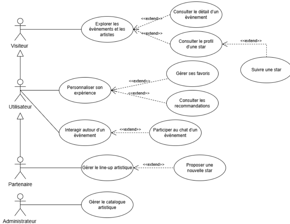
FIGURE 1.1 – Diagramme de cas d'utilisation du Sprint 3
