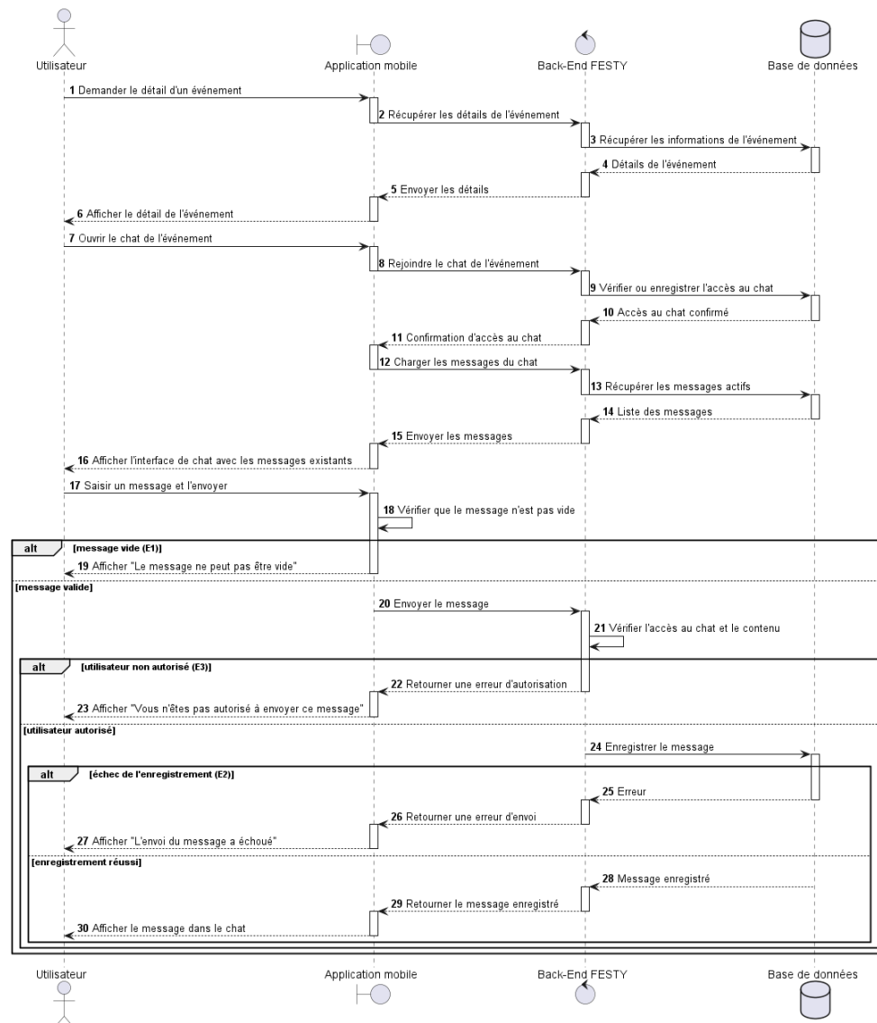
FIGURE 1.4 – Diagramme de séquence du scénario de participation au chat d'un événement
