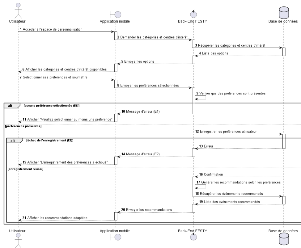
FIGURE 1.3 – Diagramme de séquence du scénario de personnalisation et recommandations
