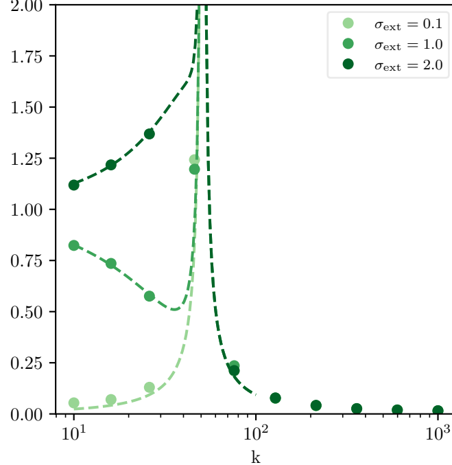
Linear Regression
