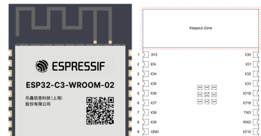
(b) Moduł WROOM [9]
