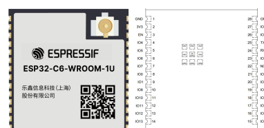
(b) Moduł WROOM [10]
