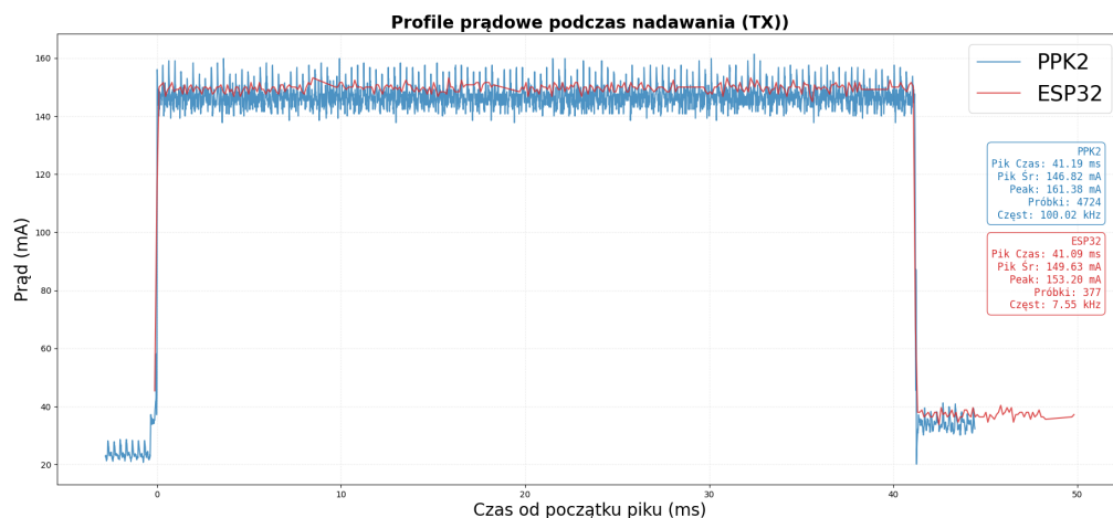
Rysunek 5.1: Porównanie profili prądowych przy nadawaniu w LoRa
