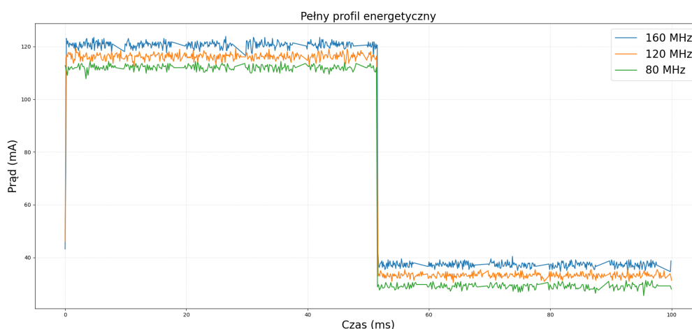
Rysunek 5.5: Porównanie profili prądowych przy różnych częstotliwościach taktowania procesora w LoRa
