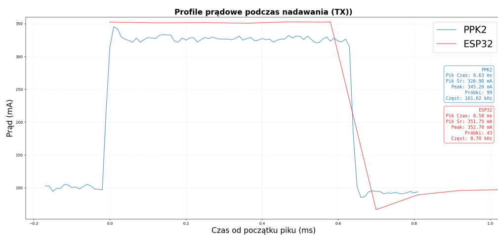
Rysunek 5.3: Porównanie profili prądowych przy nadawaniu w ESP-NOW
