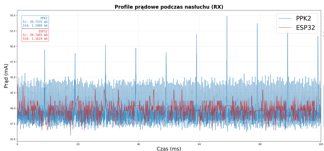
Rysunek 5.2: Porównanie profili prądowych przy nasłuchu w LoRa
