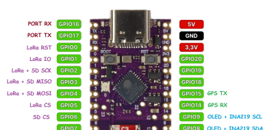
(a) Wersja deweloperska Super Mini [24]
