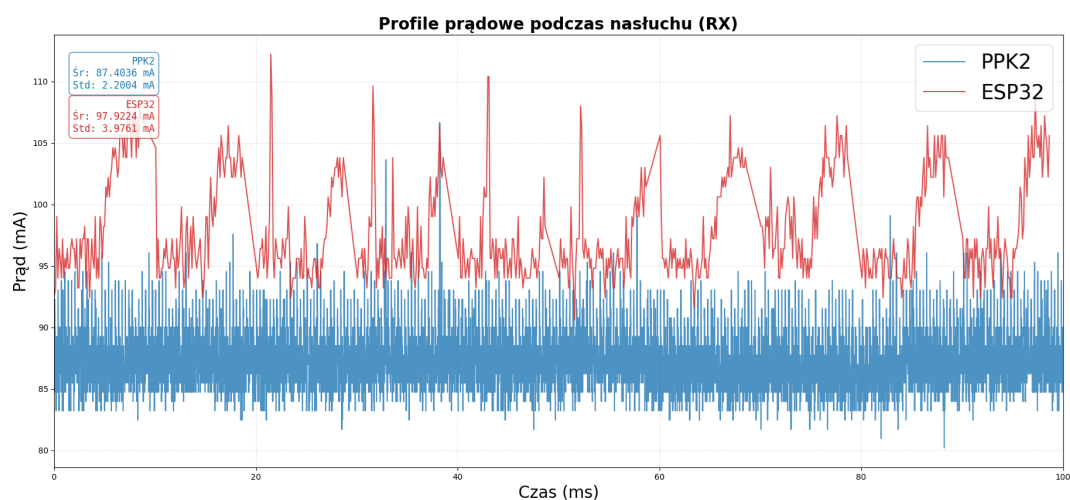
Rysunek 5.4: Porównanie profili prądowych przy nasłuchu w ESP-NOW
