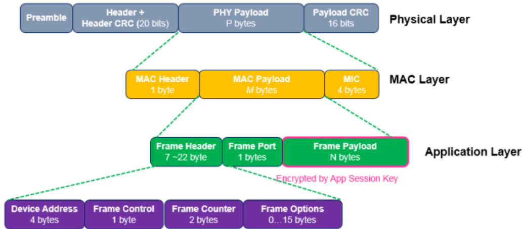
Rysunek 2.2: Struktura pakietu danych LoRa [30]
