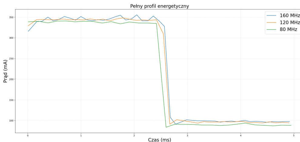
Rysunek 5.6: Porównanie profili prądowych przy różnych częstotliwościach taktowania procesora w ESP-NOW
