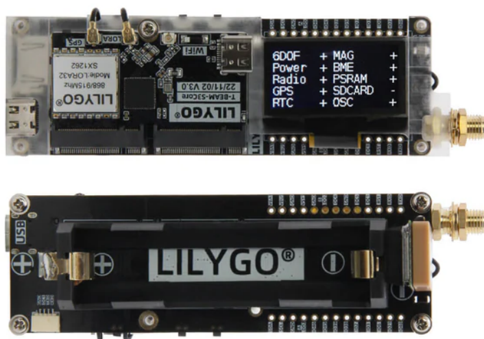
Rysunek 2.5: Moduł LILYGO T-Beam SUPREME [22]
