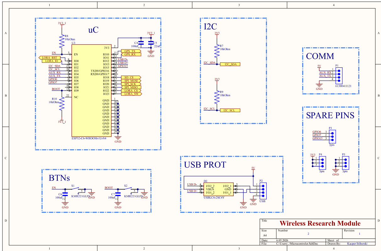
Rysunek 3.6: Schemat - Sekcja mikrokontrolera
