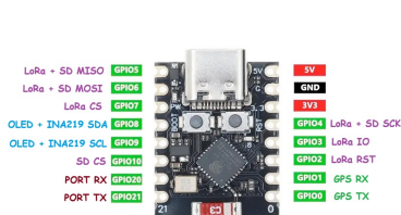
(a) Wersja deweloperska Super Mini [23]
