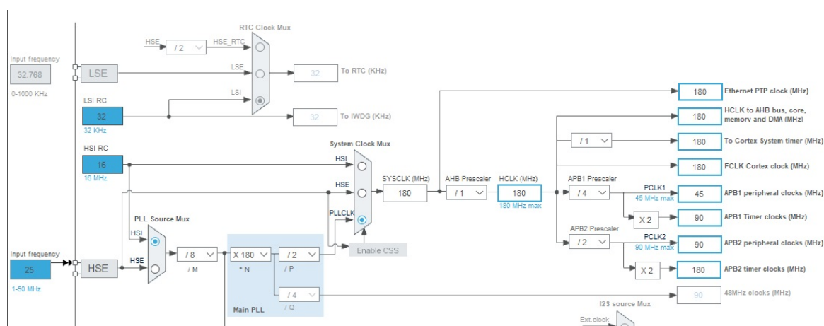
Figure 4.6. Konfiguracja sygnału zegarowego po przestawieniu HSE w tryb BYPASS
