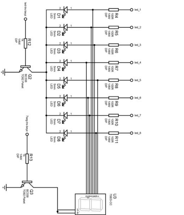
Devre Şeması
