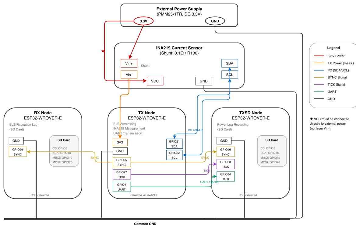
図 4.1 三ノード計測系のシステムアーキテクチャ
