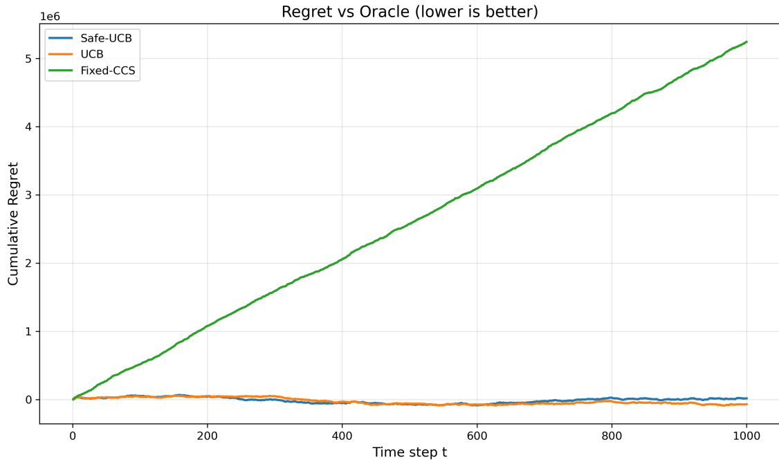
図 5.12 累積 Regret 推移 (Safe-UCB vs UCB vs Fixed-CCS)
