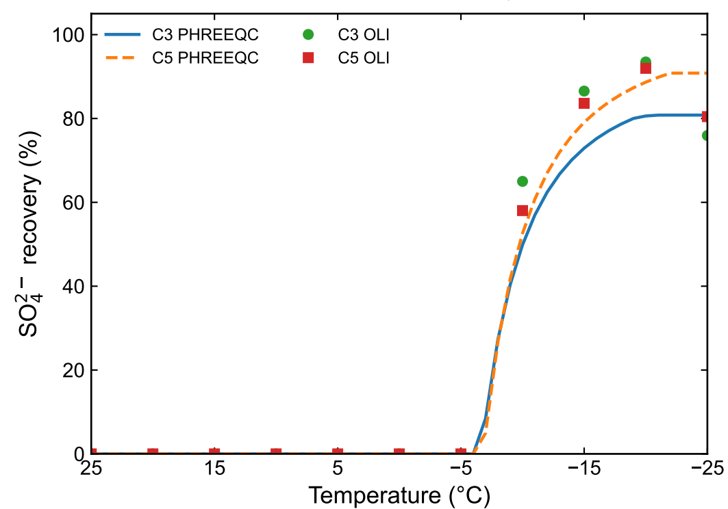
(d) Mirabilite recovery
