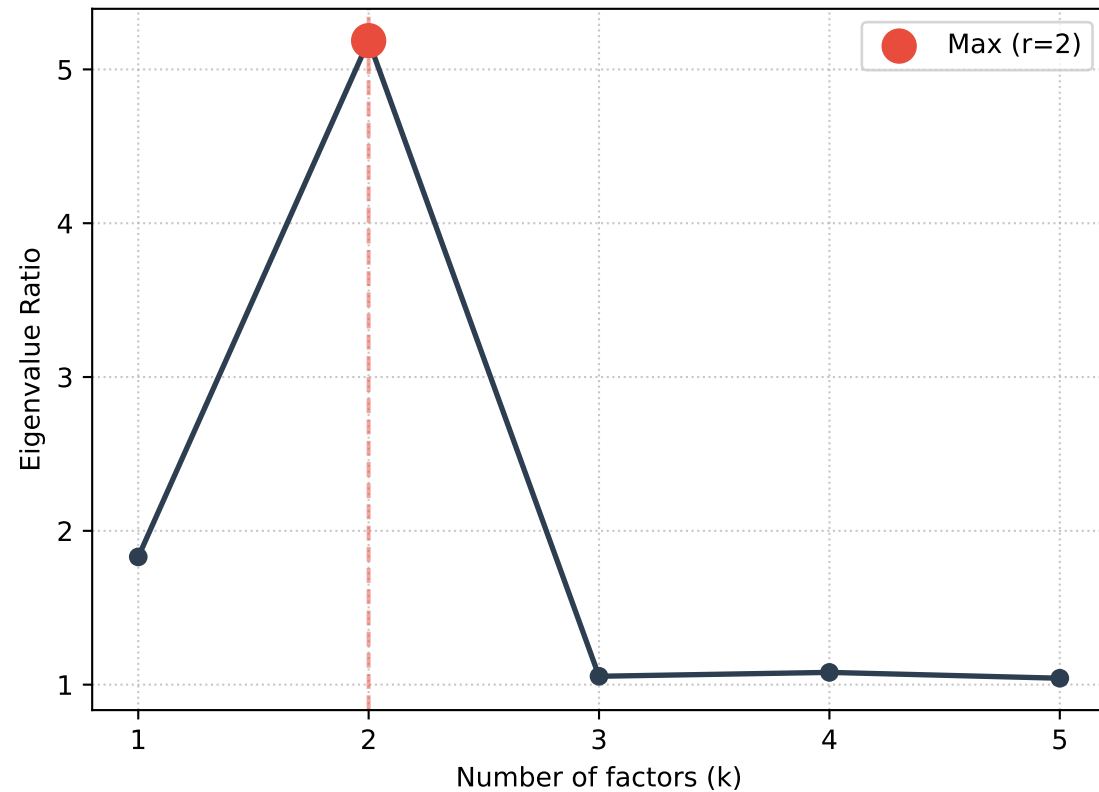
ER Criterion (Ahn & Horenstein)
