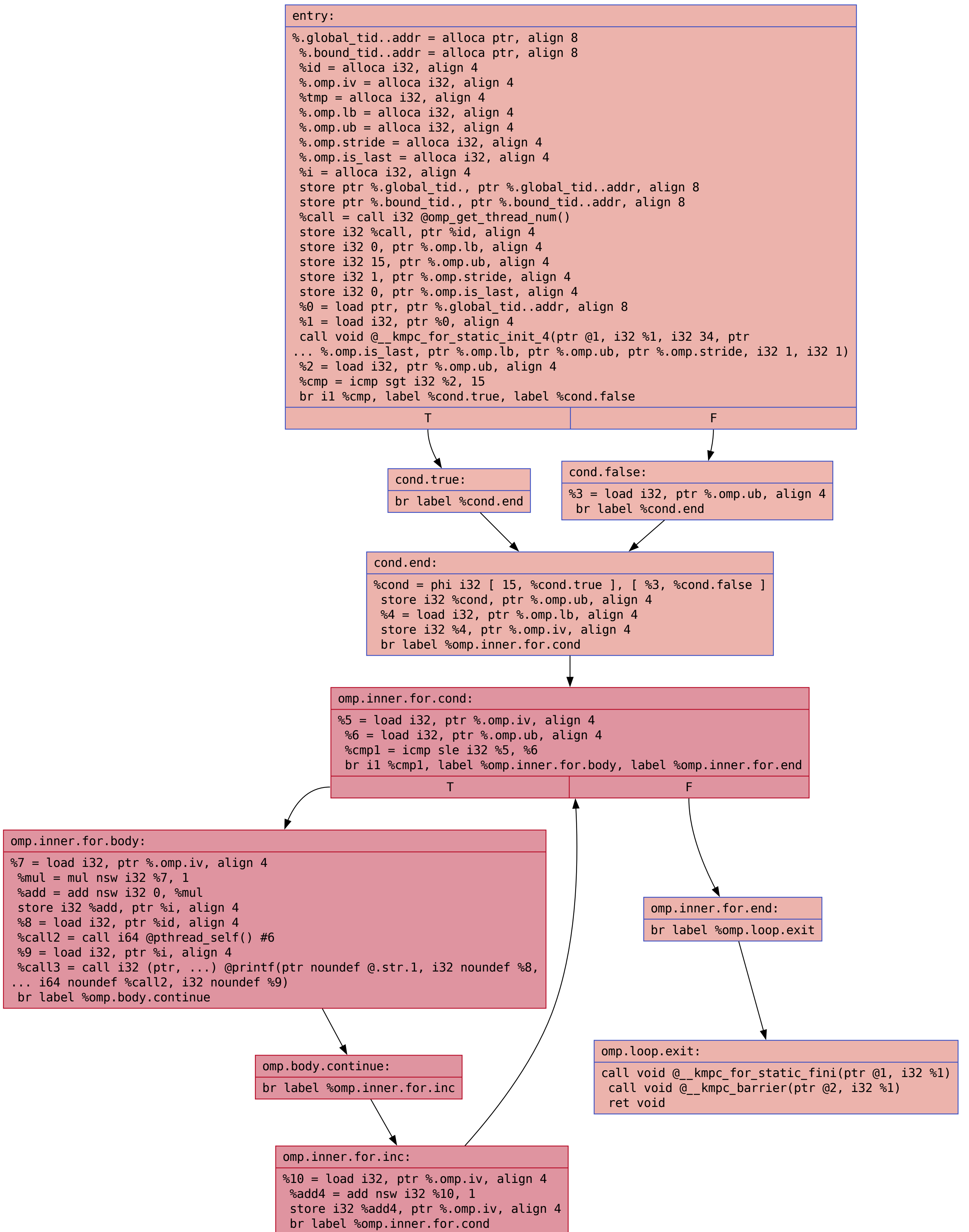
CFG for 'main.omp_outlined' function
