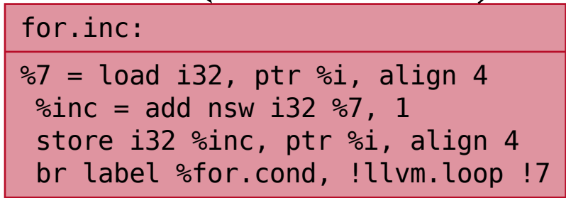
CFG for 'init_array' function
