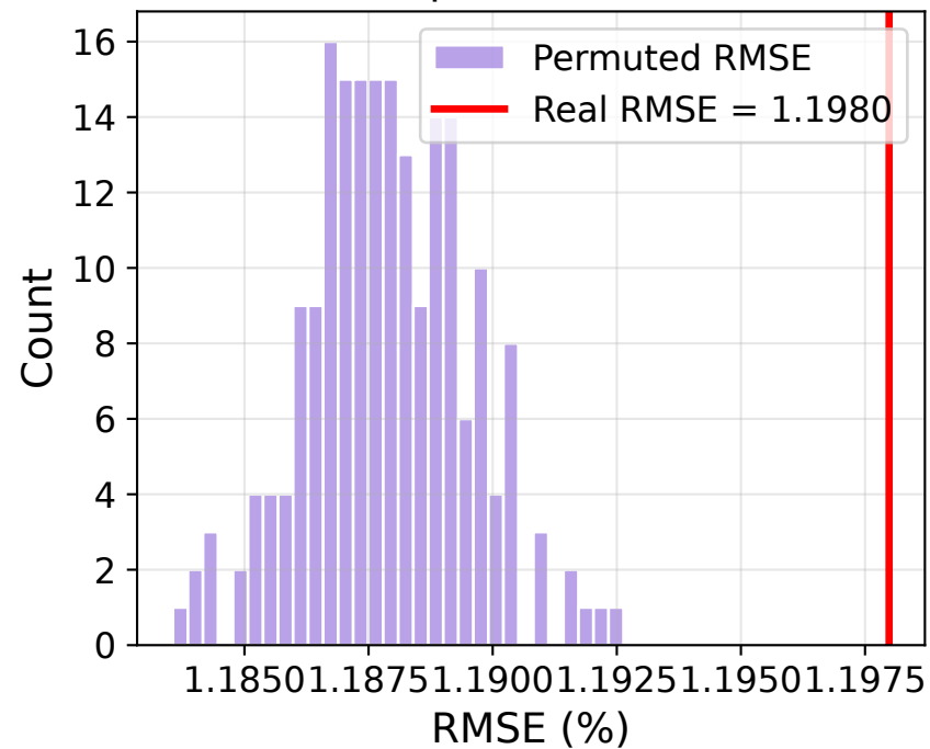
SVR p = 1.000
