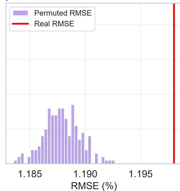
EEM - SVR p = 1.000
