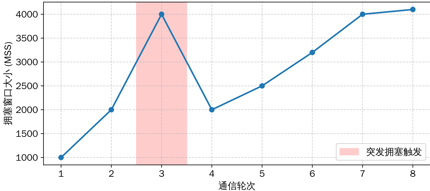
突发流量导致拥塞窗口过度减小
