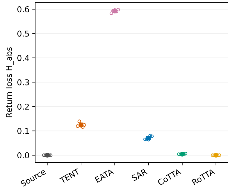
cifar100-C
