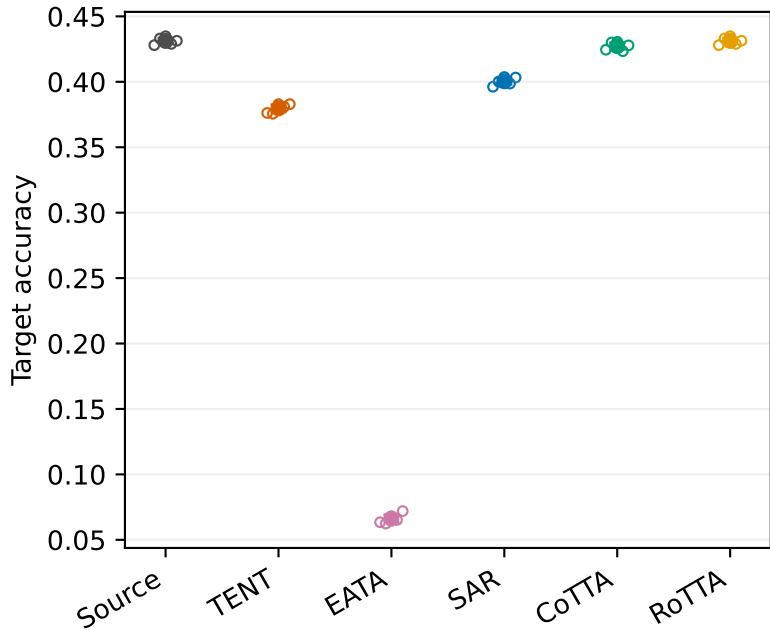
cifar100-C
