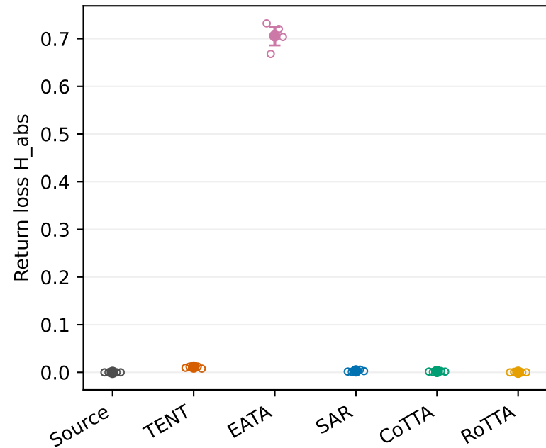
cifar10-C
