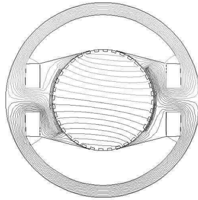
Moteur à courant continu
