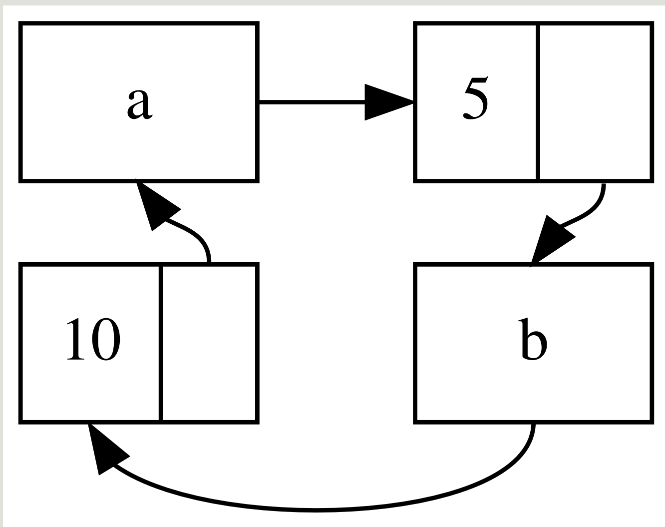
图 15-4: 列表 a 和 b 彼此互相指向形成引用循环
