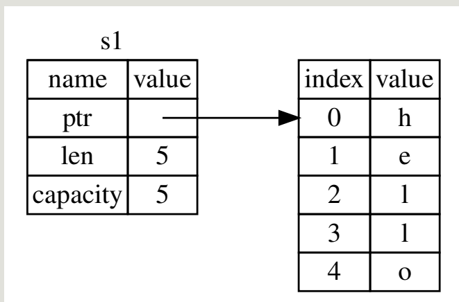
图 4-1：将值 "hello" 绑定给 s1 的 String 在内存中的表现形式
