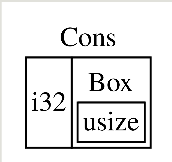
图 15-2：因为 Cons 存放一个 Box 所以 List 不是无限大小的了
