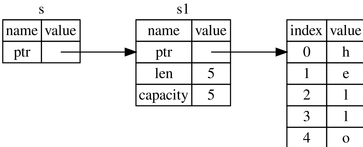
图 4-5： &String s 指向 String s1 示意图
