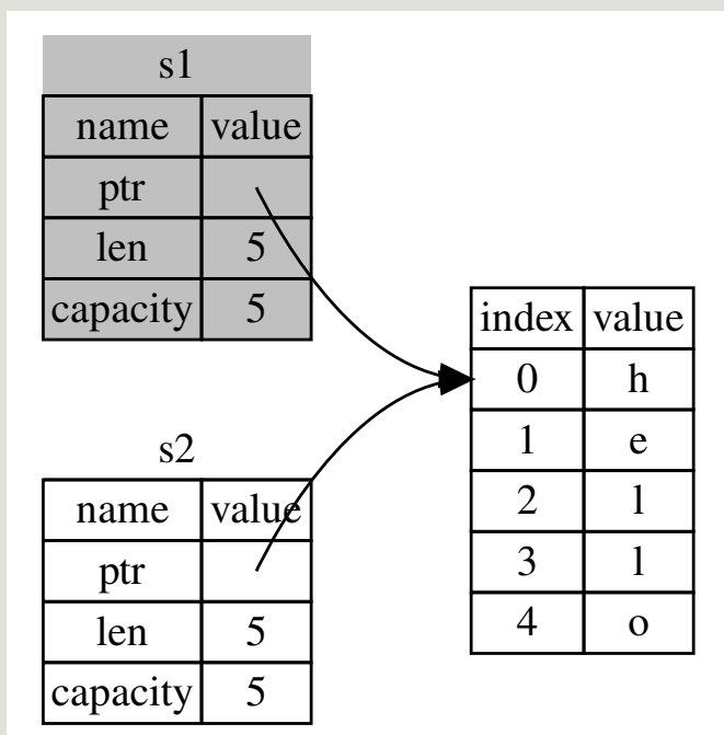
图 4-4： s1 无效之后的内存表现
