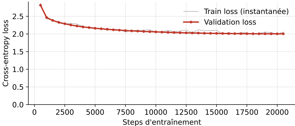
Évolution de la loss (Chat Musicien, 2 epochs sur Tesla T4)
