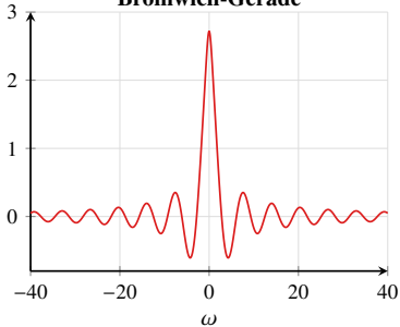
Bromwich-Gerade
