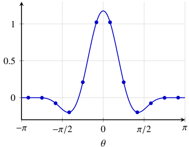
Talbot-Kontur
