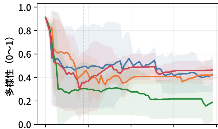
Airfoil：集団多様性
