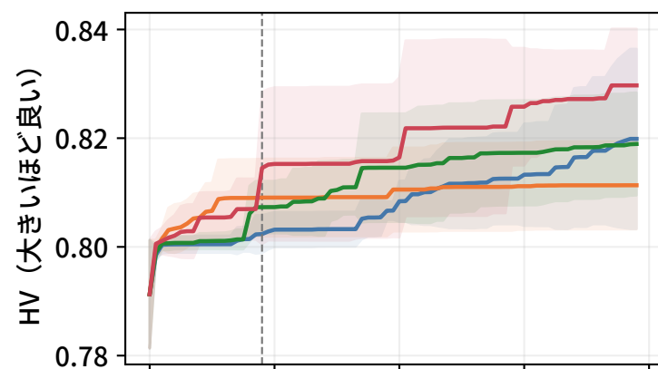
Concrete：アーカイブHV
