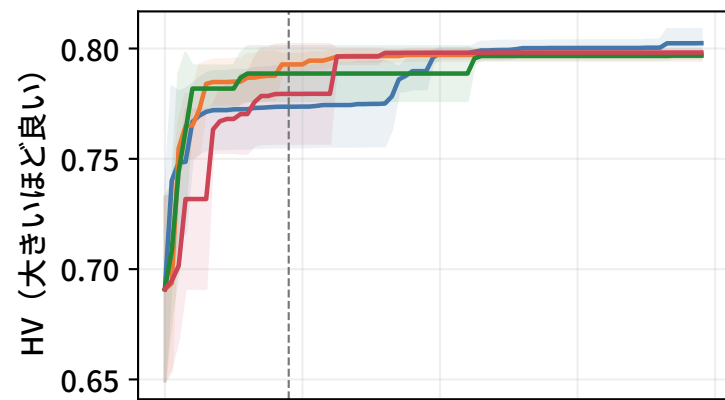
Airfoil：アーカイブHV
