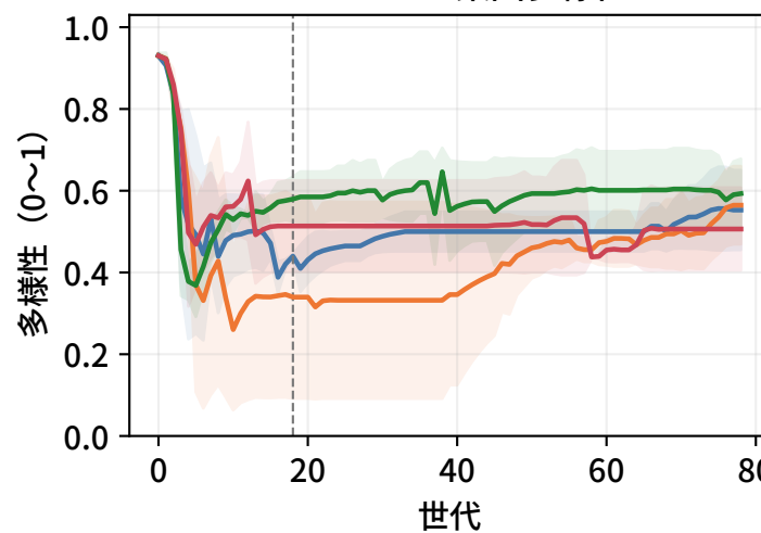
Concrete：集団多様性
