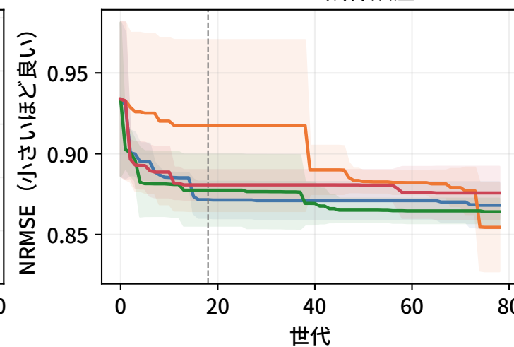
Concrete：訓練誤差
