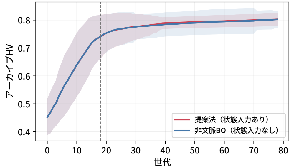
アーカイブHVの推移
