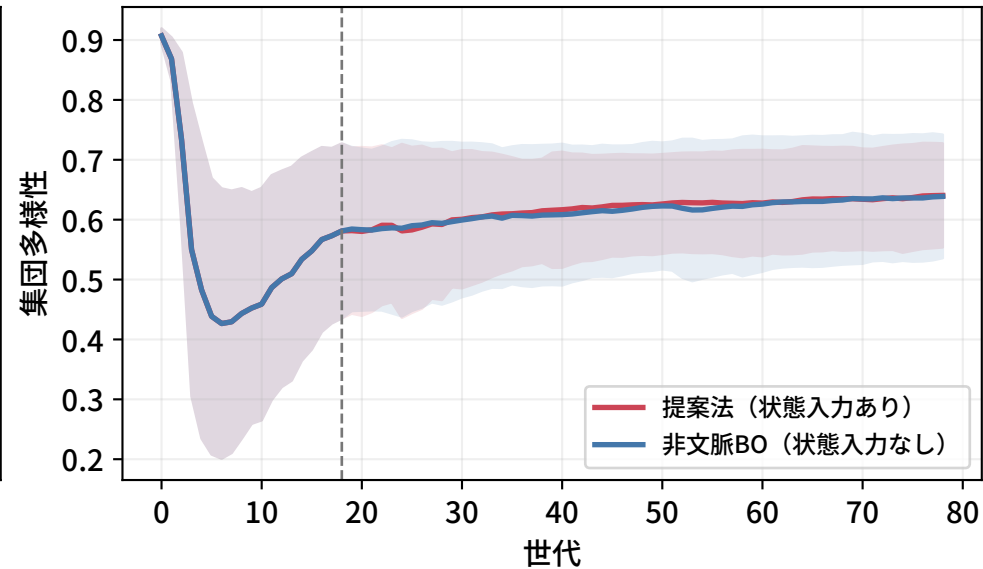
集団多様性の推移
