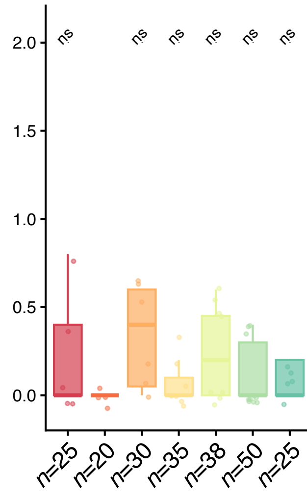
Corynebacteriaceae
