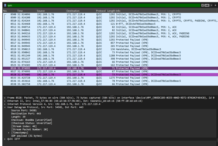
Рис. 2.21: Исходящий quic пакет
