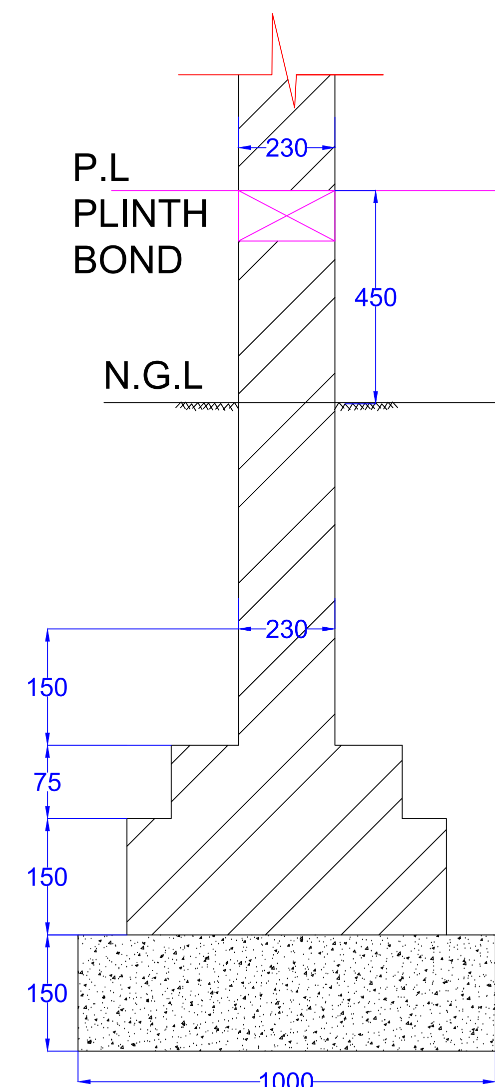
FOUNDATION DETAIL N.T.S
