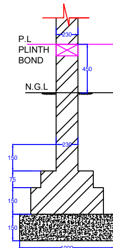
FOUNDATION DETAIL N.T.S
