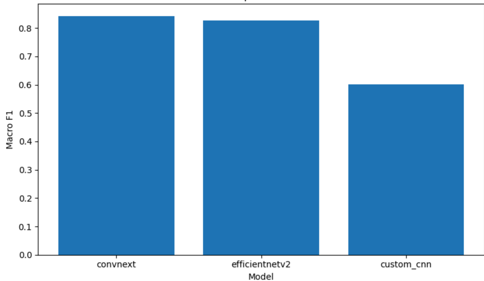
Model Comparison: Macro F1
