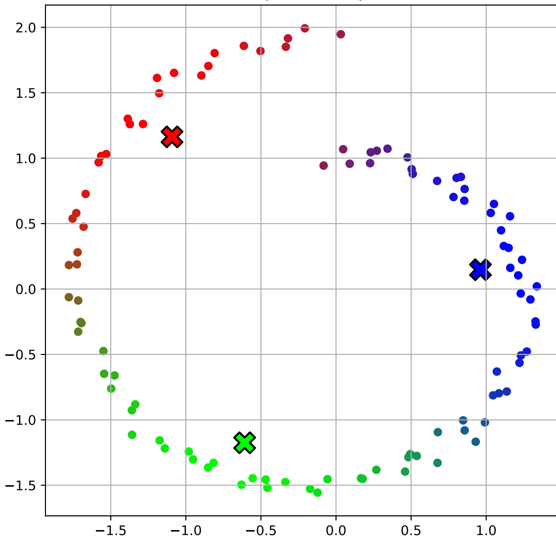
FCM - po 20 iteracjach
