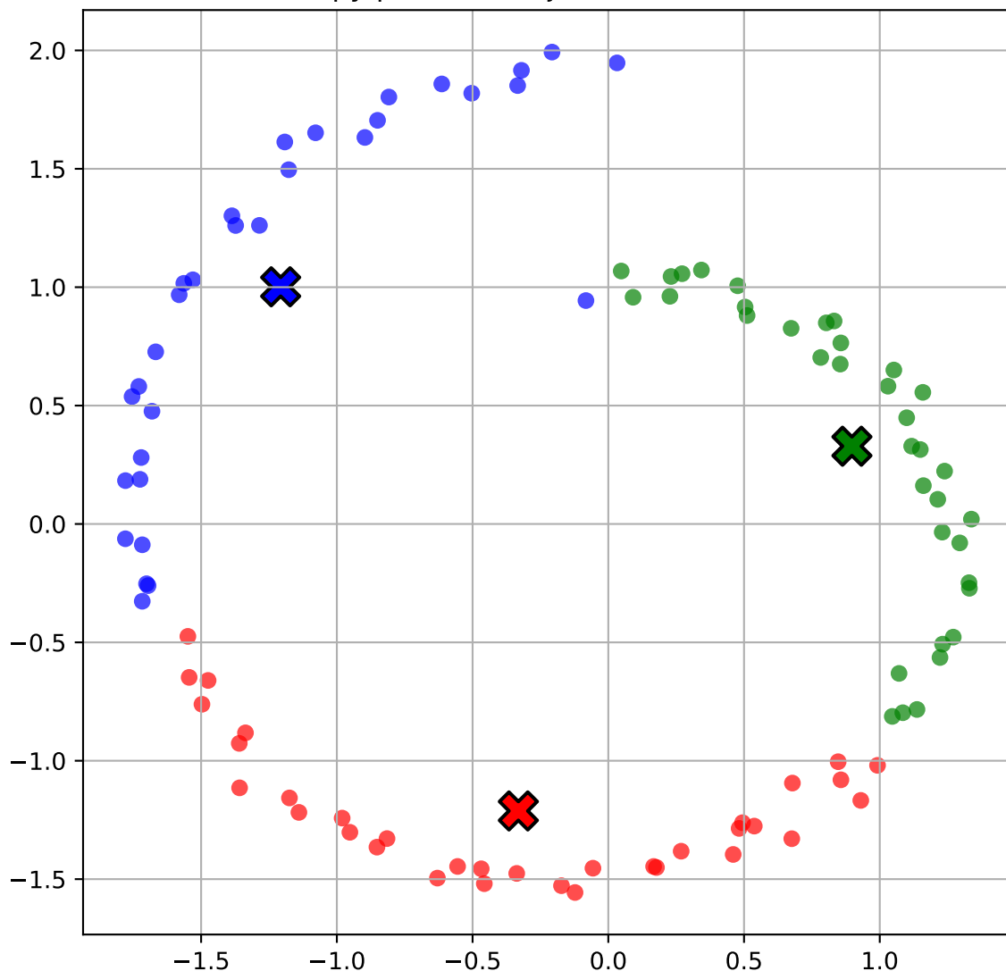
Grupy po 10 iteracjach - euklidesowa
