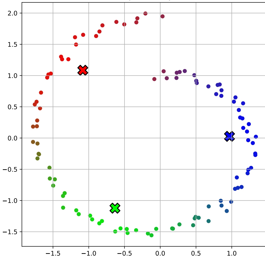
FCM - po 4 iteracjach
