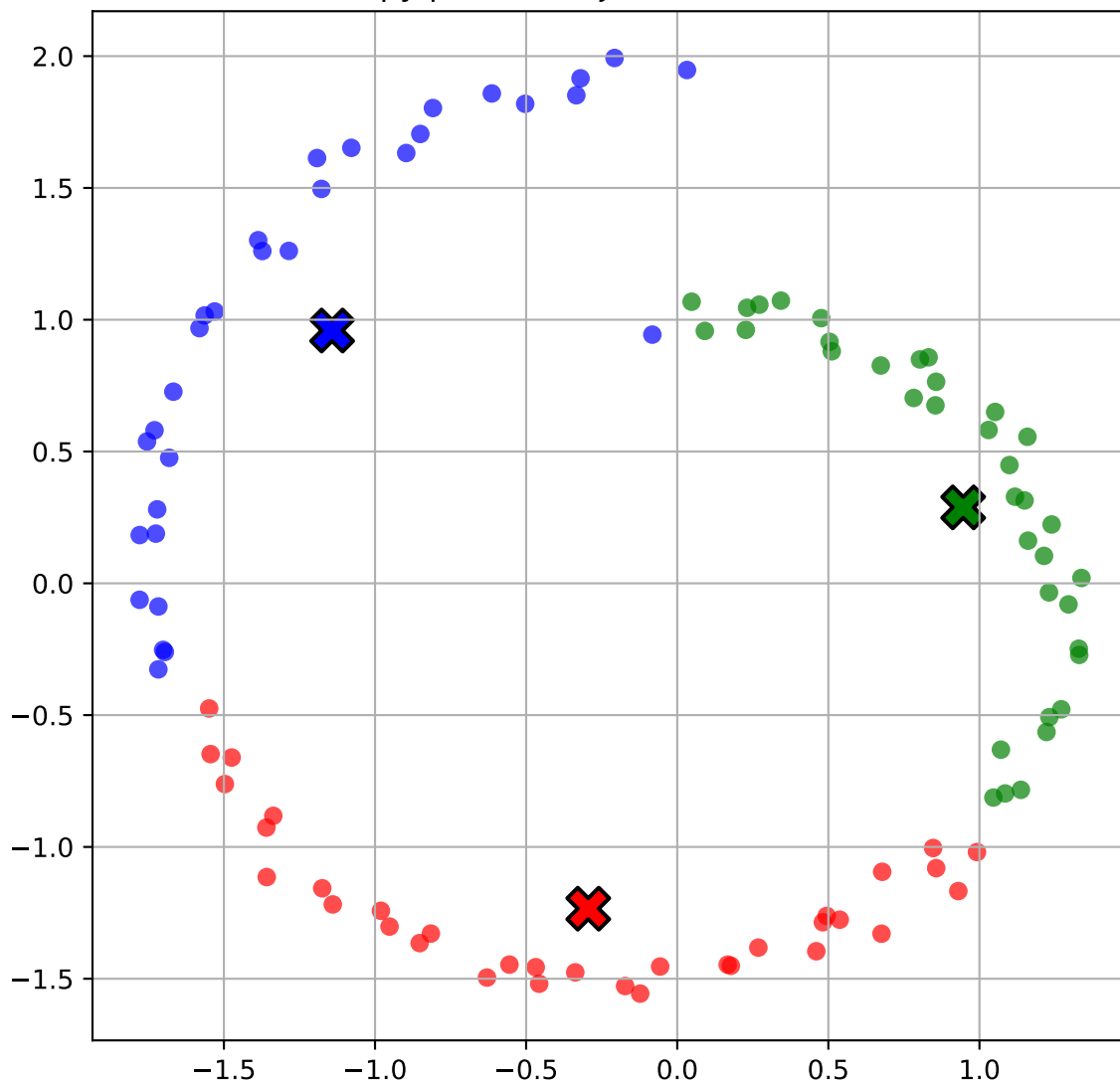
Grupy po 4 iteracjach - euklidesowa
