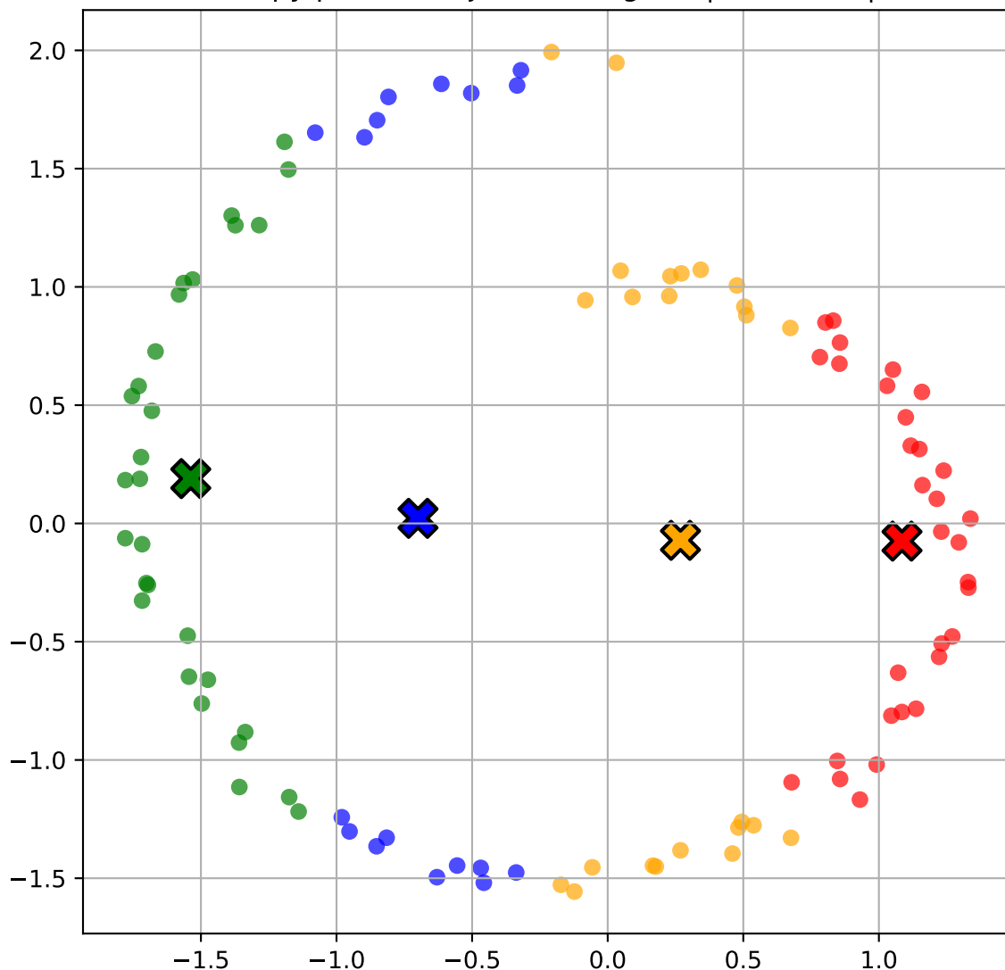
Grupy po 4 iteracjach - odległość |x_{1A} - x_{1B}|
