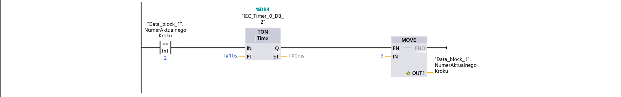
Network 11: Krok 4 - A czerwone, B czerwone
