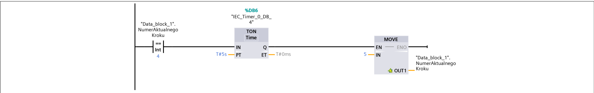
Network 13: Krok 6 - A czerwone, B zielone
