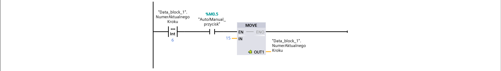
Network 23: Krok 16 Manual - A czerwone, B żółte
