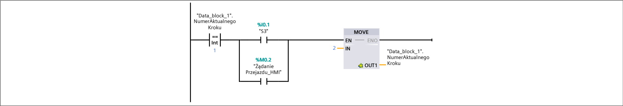
Network 10: Krok 3 - A żółte, B czerwone
