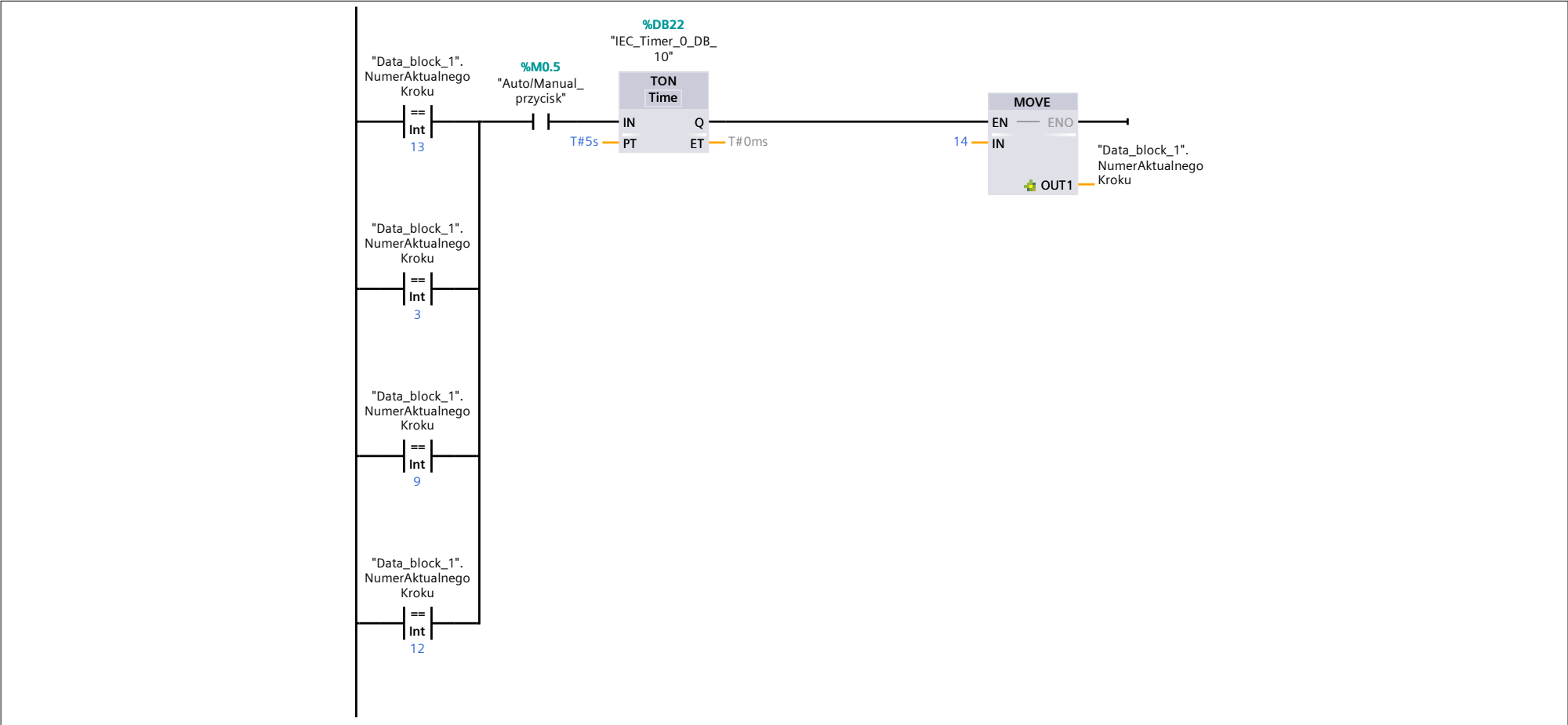
Network 22: Krok 15 Manual - A czerwone, B zielone
