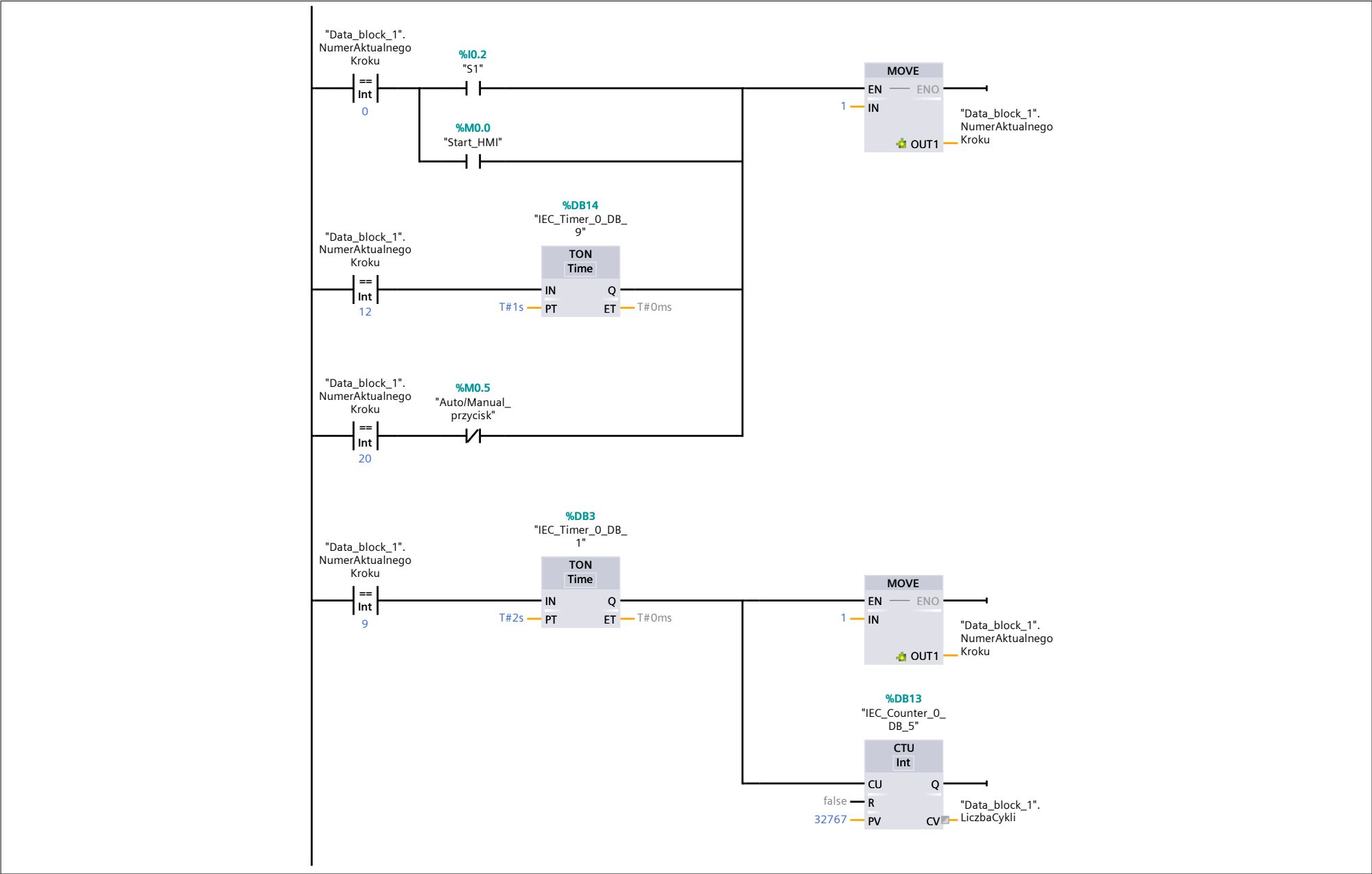
Network 9: Krok 2 - A zielone, B czerwone
