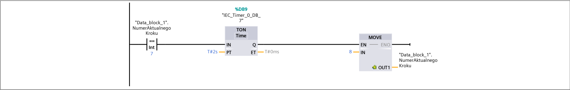
Network 16: Krok 9 - A czerwone i żółte, B czerwone
