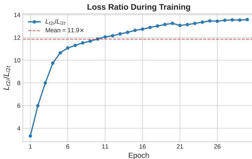
图 2: 训练期间原始（未加权）文本-图像损失与图像-文本损失的比值 L_{t2i}/L_{i2t} ( \alpha=0.75 )。尽管存在偏向 t2i 的显式优化偏差，该比率从第一个周期的约 3.3 倍上升到收敛时的超过 13.5 倍，均值为 11.86 倍（虚线）。这一不断扩大的差距表明队列引发的非对称性主导了损失重加权的效应。
