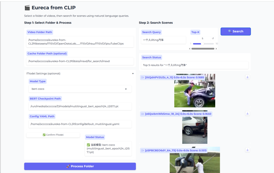
图 3: 多语言检索实例：查询”一个人 lifting 汽车”。模型检索到人抬起汽车的视频片段，展示了中英文混合查询下跨语言词汇的联合匹配能力。
