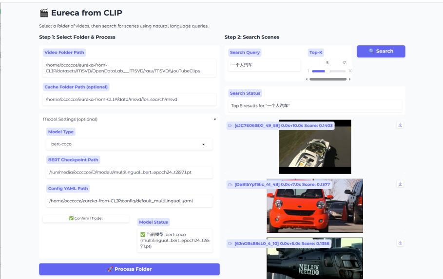
图 4: 多语言检索实例：查询”一个人汽车”。模型检索到一个人驾驶汽车的视频片段。结合图3，加入英文词”lifting” 后检索结果切换为抬起汽车，展示了模型对中英文混合查询的灵活处理能力。
