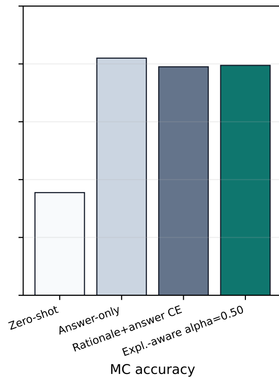
Qwen2-VL / A-OKVQA
