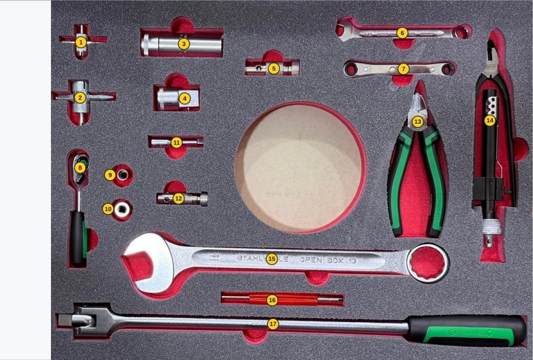
SCANAEROTECH SCA-SAS321-010
