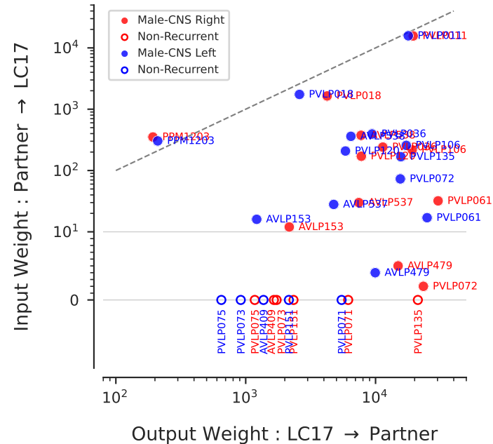
Male-CNS
