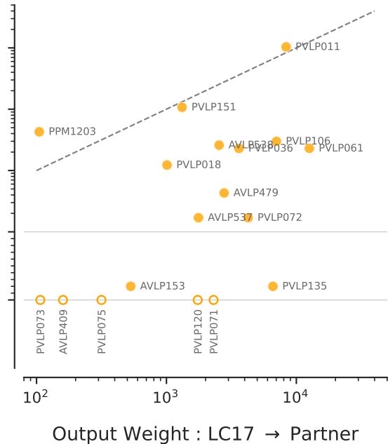
Hemibrain
