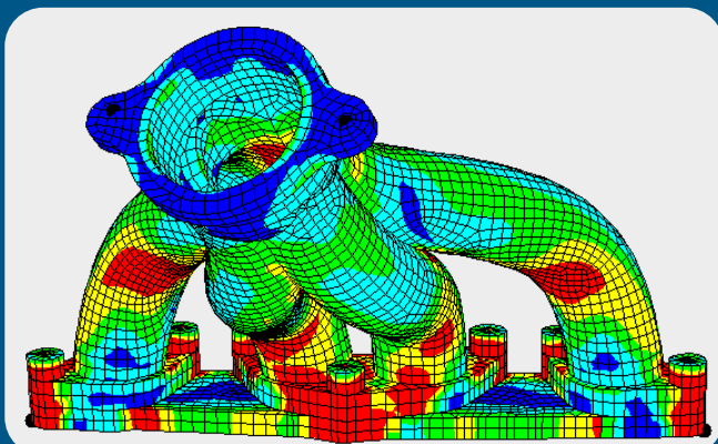
弹塑性铸铁
