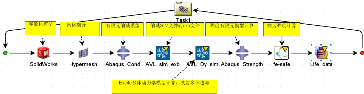
CAD、MESH、FEA、MBD、Fatigue自动化集成仿真
