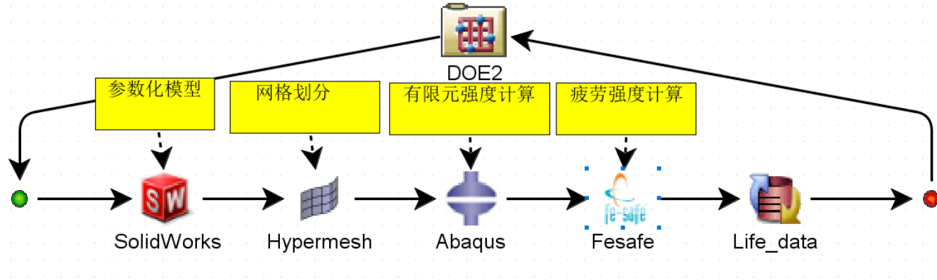
CAD、MESH、FEA、Fatigue自动化集成仿真
