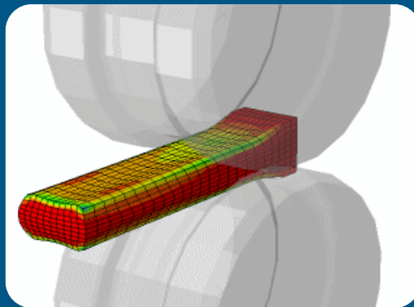
金属轧制
