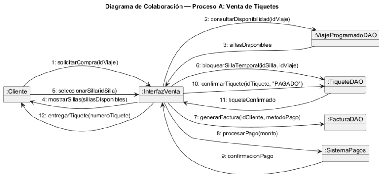
Figure 9: Diagrama de colaboración — Proceso A: Venta de Tiquetes
