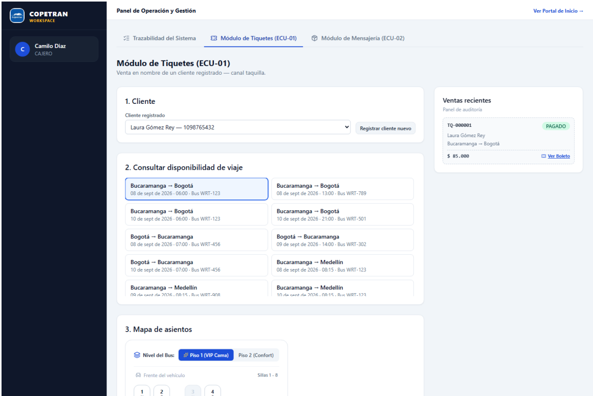
Figure 16: Módulo de Tiquetes — mapa de asientos interactivo (RF01, RF03)
