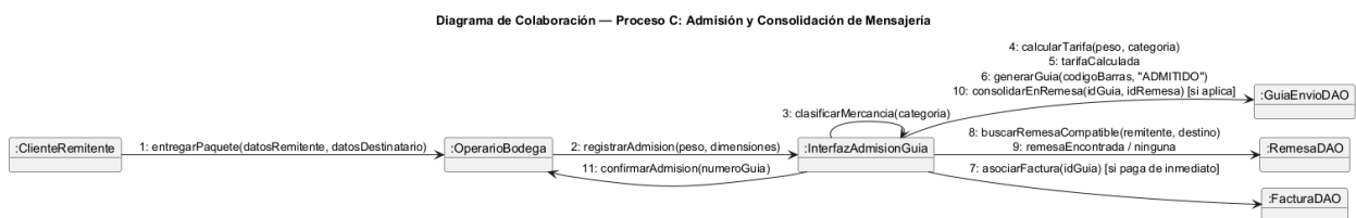
Figure 10: Diagrama de colaboración — Proceso C: Admisión y Consolidación de Mensajería
