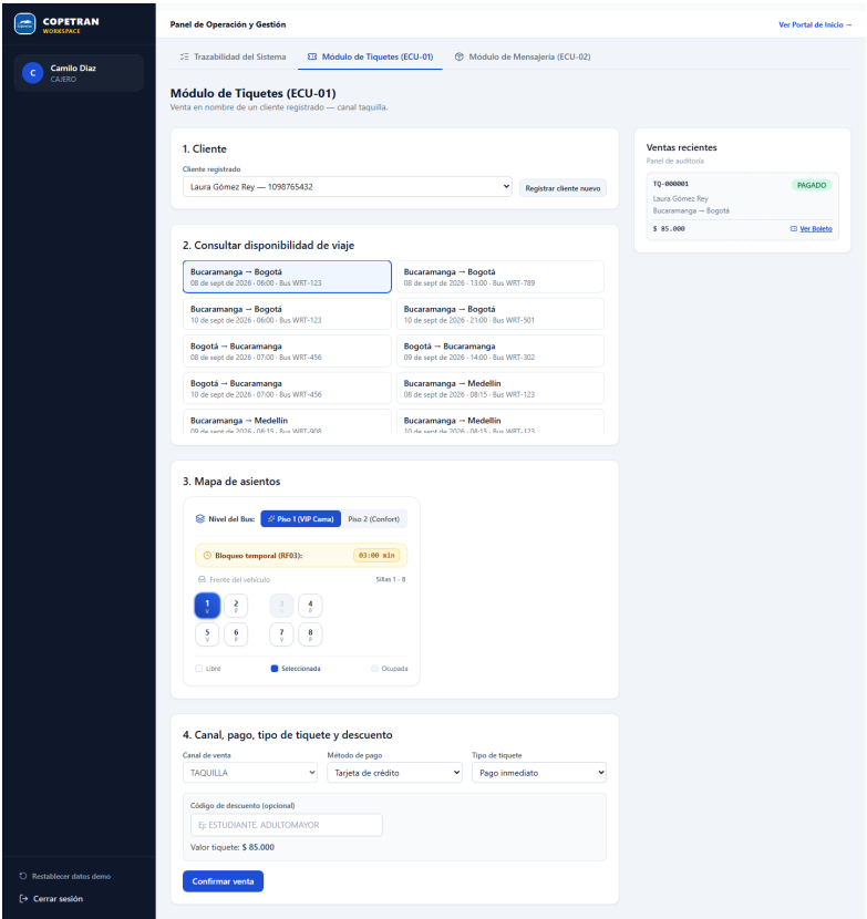
Figure 17: Evidencia puntual de RFO3: al seleccionar la silla 1 se activa el temporizador regresivo de bloqueo temporal (03:00 min, cuenta en tiempo real cada segundo)
