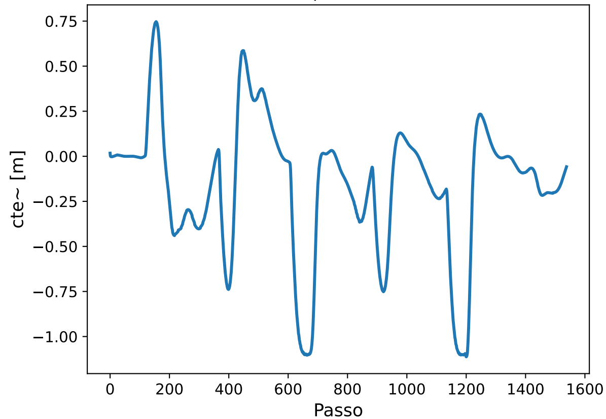
Erro lateral (aprox) - Pure Pursuit
