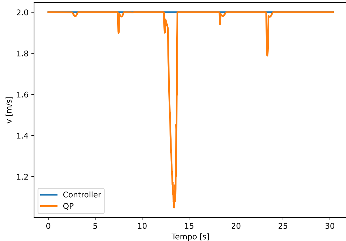
Velocidade linear: Controller vs QP
