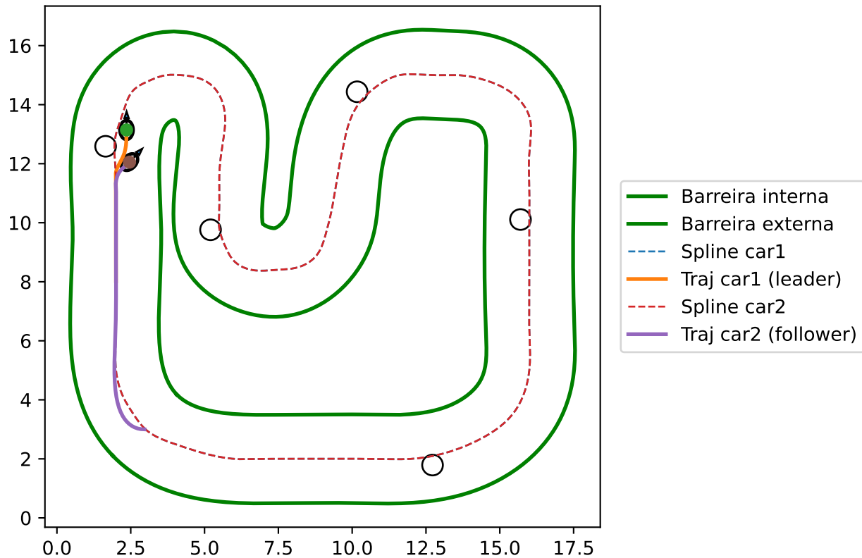
Multi-carro: Pure Pursuit + CBF-QP (caminho do simulate1)
