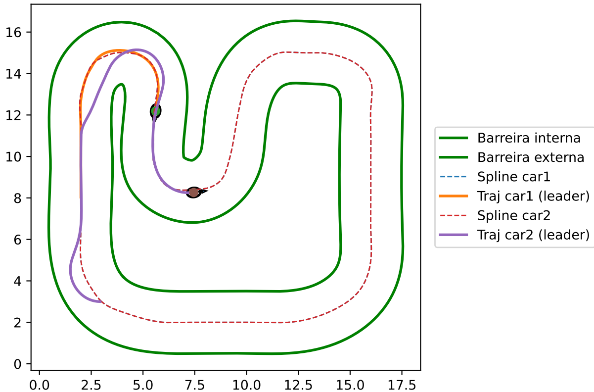
Multi-carro: Pure Pursuit + CBF-QP (caminho do simulate1)
