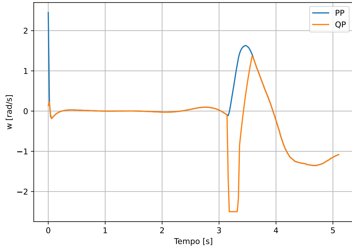
Velocidade angular: PP vs QP
