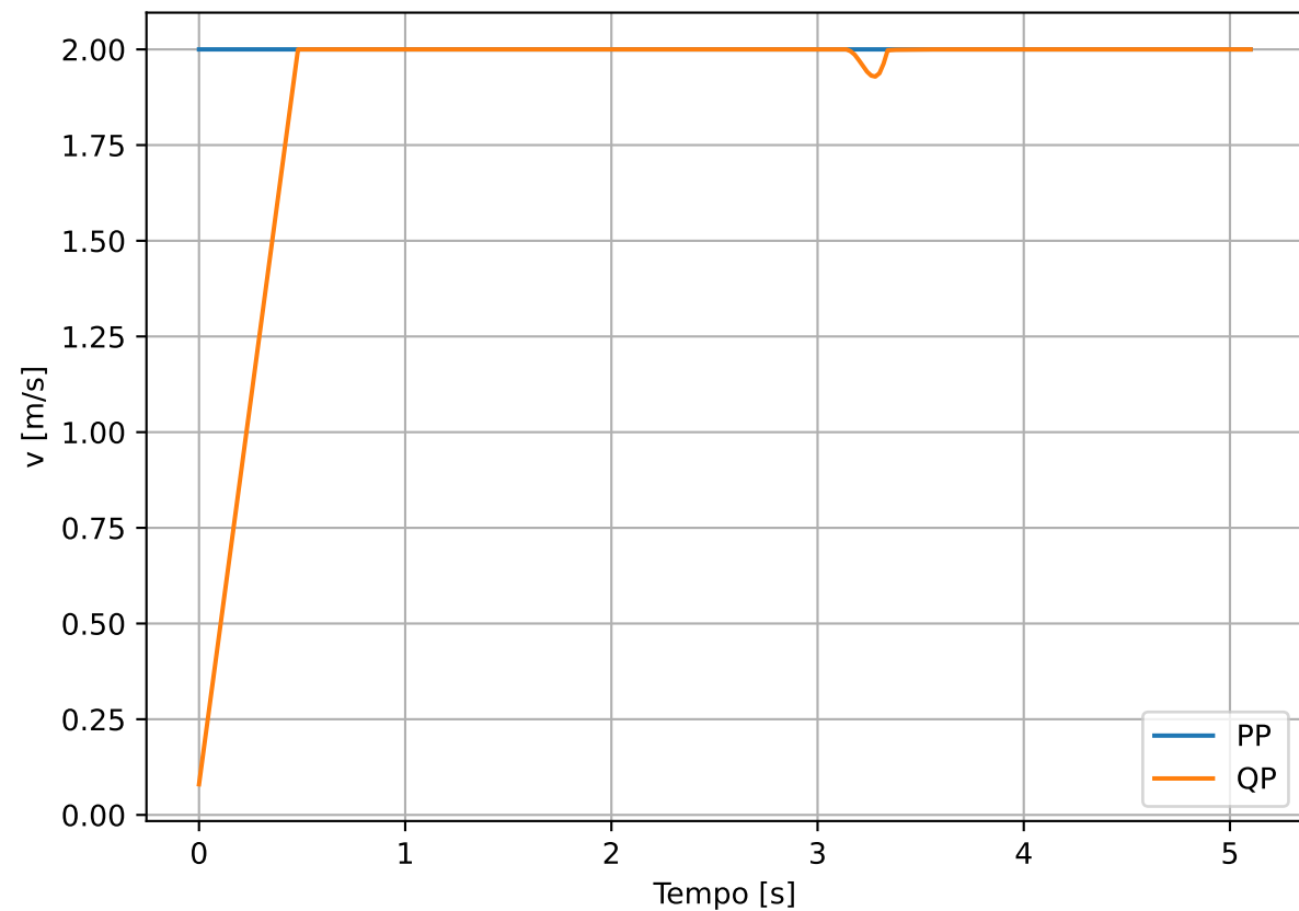
Velocidade linear: PP vs QP
